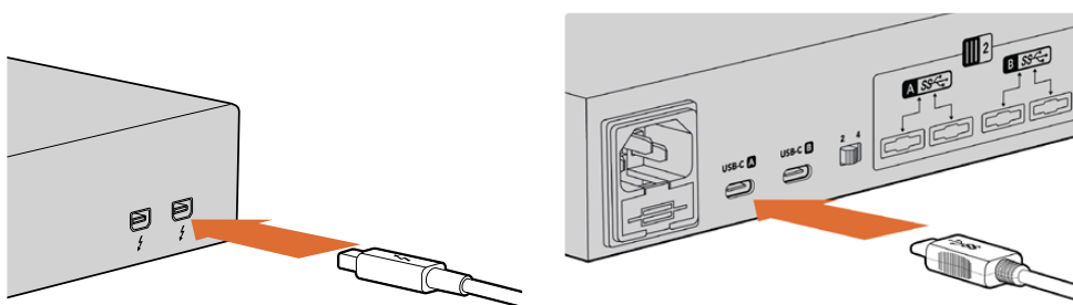
Branchez le Blackmagic MultiDock à votre ordinateur Mac ou PC Windows à l'aide d'un câble Thunderbolt ou USB-C.
